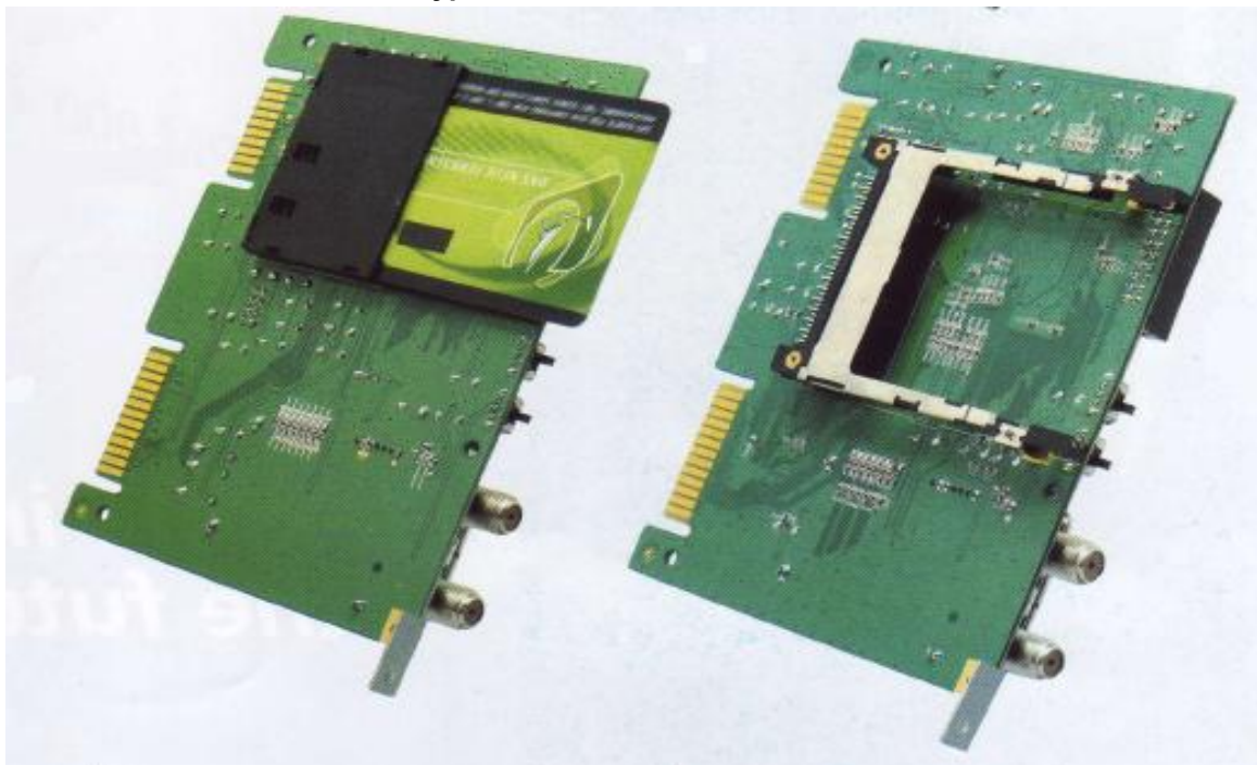
Modulátor
